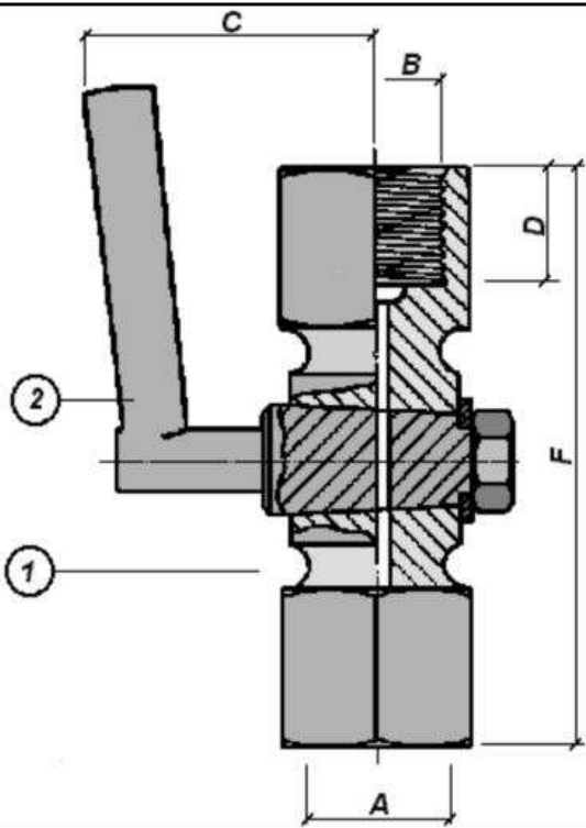
GRIFO MANOMETRO FIG. 226
